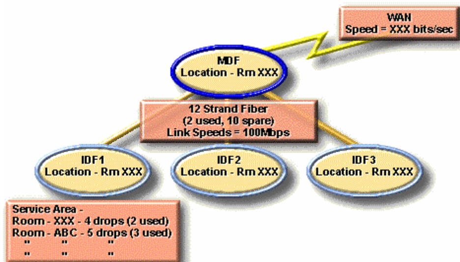
Hình 7.6 – Tài liệu về dây nối tại một IDF
