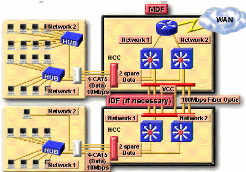
Hình 7.15 – Sử dụng router để phân chia vùng dụng độ trong mạng
