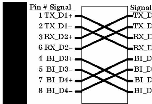
Hình 2.14 – Sơ đồ bấm dây cho chuẩn mạng 100 BASE-T4
