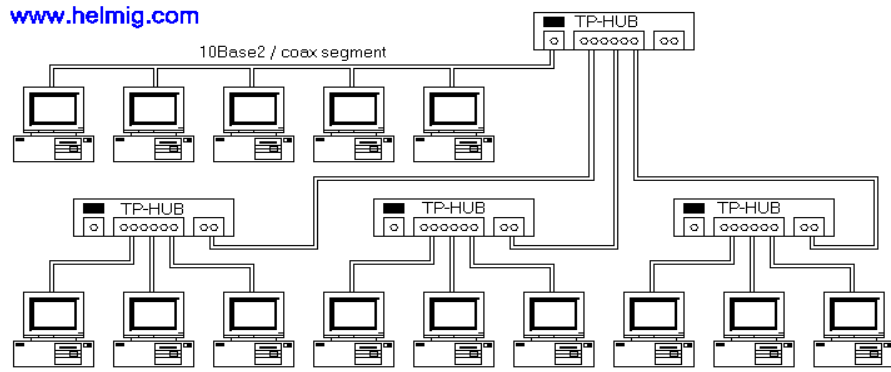
Hình 2.11 – Sử dụng HUB để nối nhiều HUB
