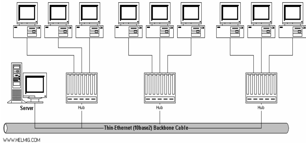
Hình 2.12 – Nối kết các HUB bằng cáp đồng trục gầy
