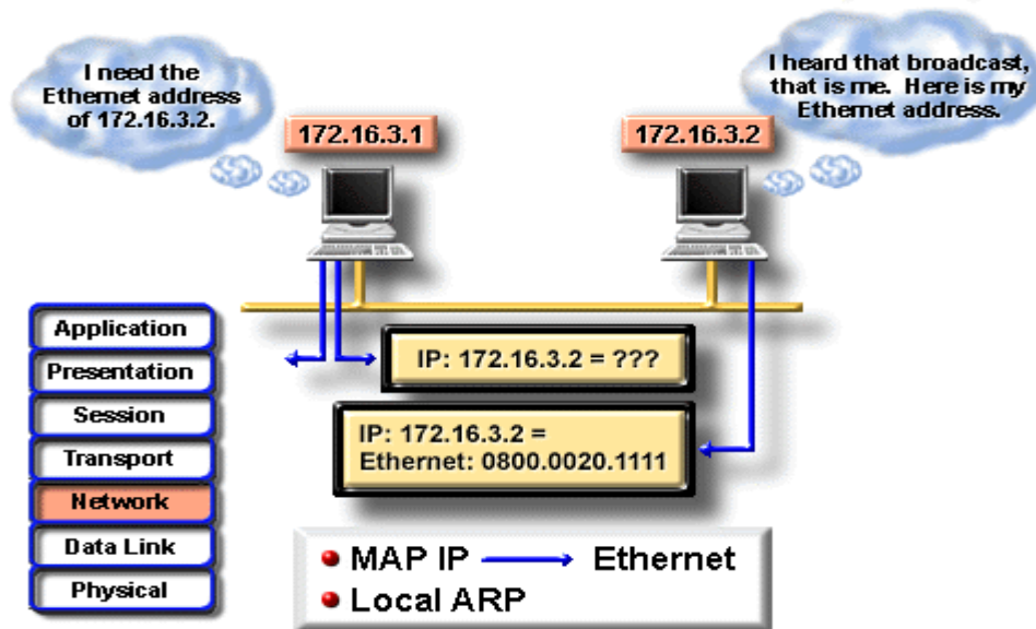
Hình 5.10 – Giao thức ARP
