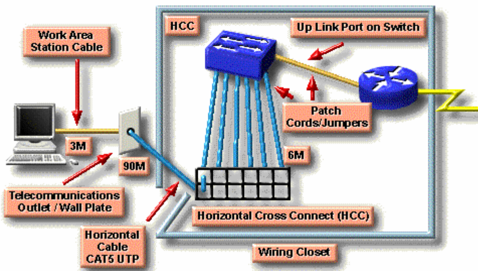
Hình 7.1 – Sử dụng MDF cho các mạng có đường kính nhỏ hơn 200 mét
