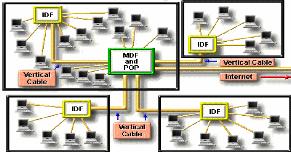
Hình 7.3 – Sử dụng thêm các IDF cho các mạng có đường kính lớn hơn 200 mét
