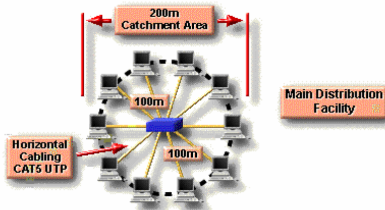
Hình 7.2 – Sử dụng HCC patch panel trong MDF
