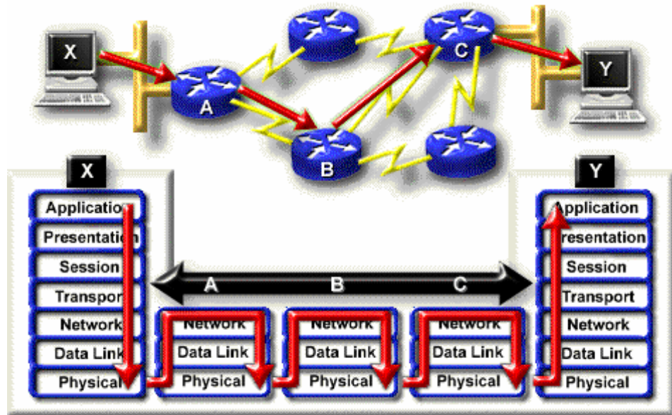
Hình 5.4- Đường đi của một gói tin qua liên mạng
