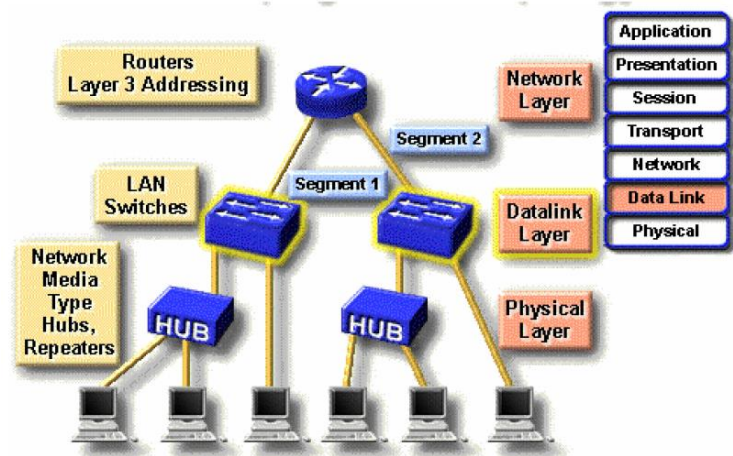
Hình 7.7 – Sử dụng Switch để mở rộng băng thông mạng
