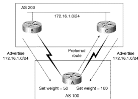
Hình 5.14 – Sử dụng thuộc tính weight trong BGP
