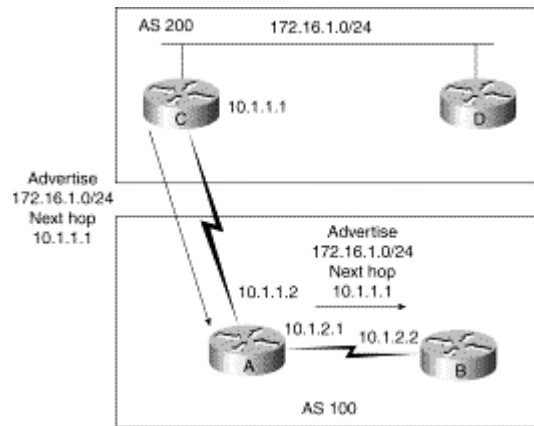
Hình 5.18 – Sử dụng thuộc tính Next-Hop trong BGP
