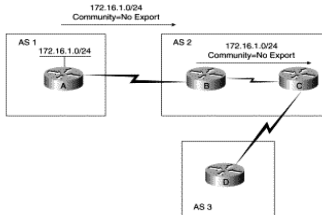
Hình 5.20 – Sử dụng thuộc tính no-advertise trong BGP
