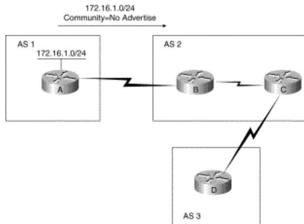
Hình 5.21 – Sử dụng thuộc tính Internet trong BGP
