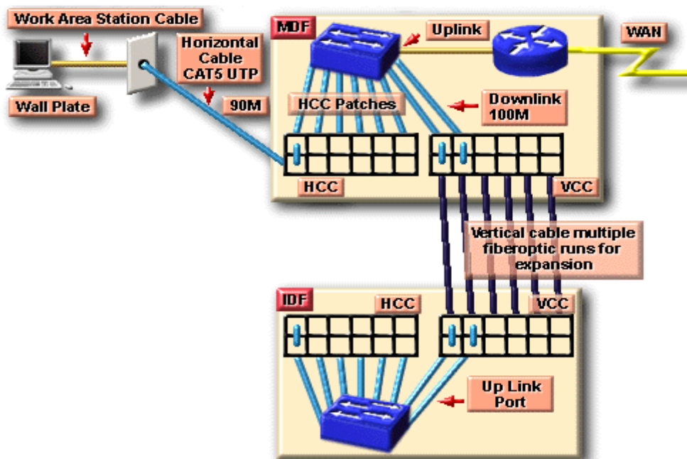
Hình 7.4 – Sử dụng VCC patch panel để nối IDF với MDF
