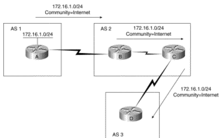
Hình 5.19 – Sử dụng thuộc tính community trong BGP
