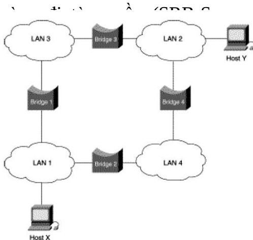
Hình 3.6 – Cầu nối trong mạng Token Ring
