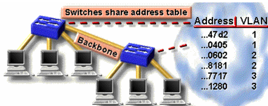
Hình 6.1 – VLAN sử dụng cơ chế lọc khung
