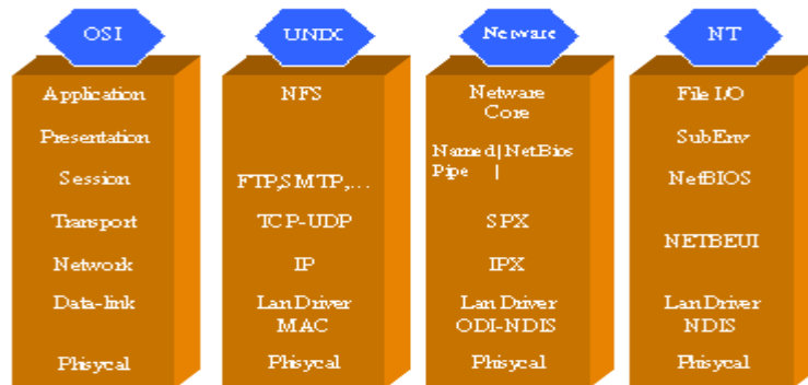
Hình 1.1 - Kiến trúc của một số hệ điều hành mạng thông dụng
