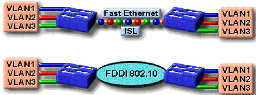
Hình 6.8 - Thiết kế VLAN xuyên qua Backbone
