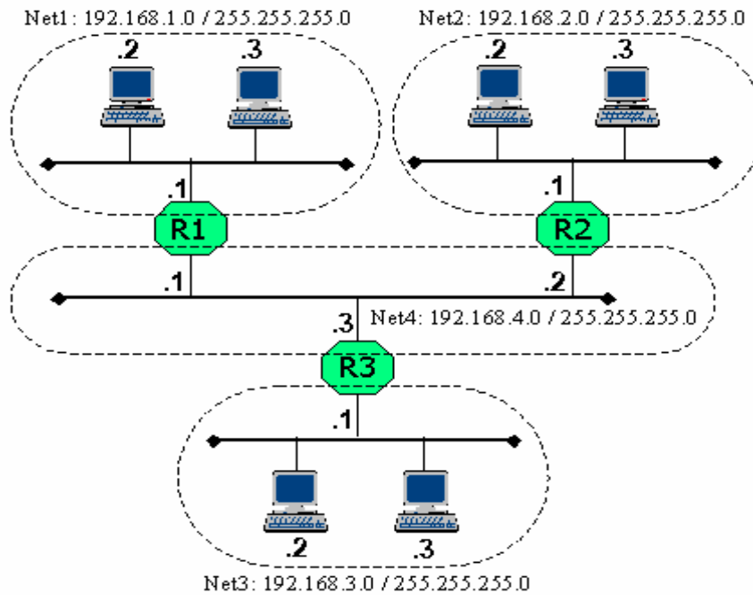
Hình 5.7 – Liên mạng sử dụng giao thức IP
