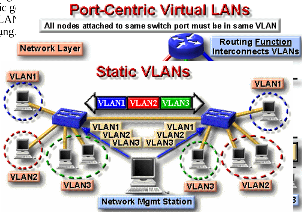
Hình 6.5 – Cài đặt VLAN dựa trên cổng
