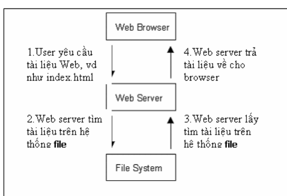
Hình 21.3: Sơ đồ hoạt động của Web Server .
