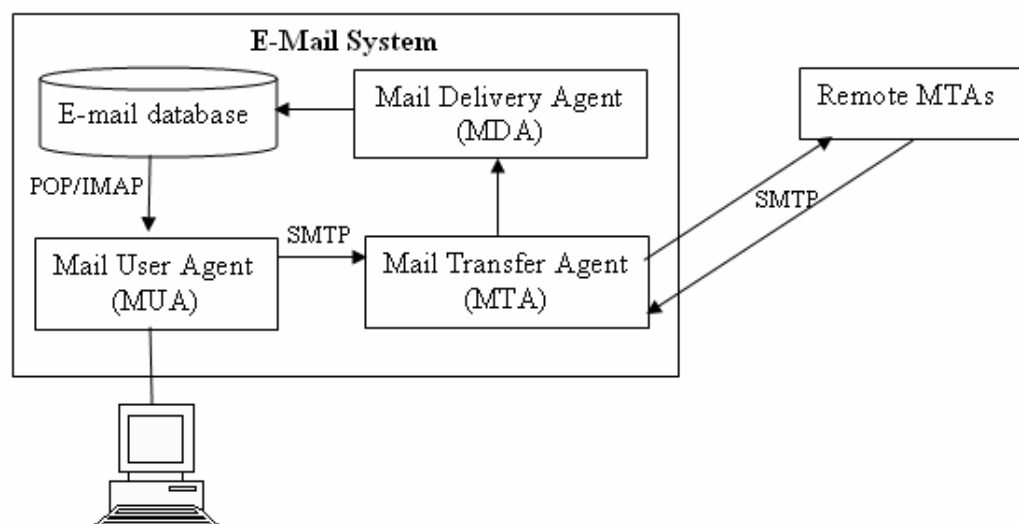
Hình 1.2. Sơ đồ tổng quan hệ thống thư điện tử Chúng ta sẽ dần dần tìm hiểu kỹ các nhân tố này.
