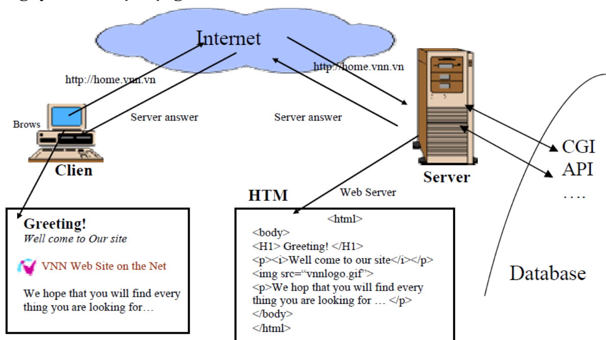
Hình 21.2: Sơ đồ hoạt động của WebServer
